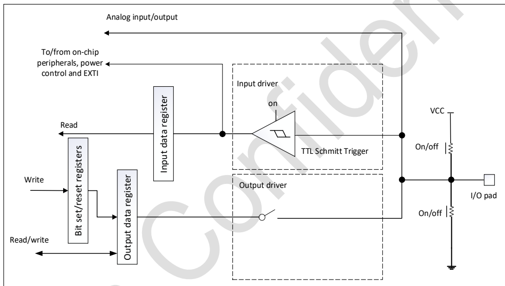
图 8-2 输入浮空/上拉/下拉配置
