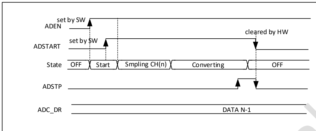
图 12-5 停止时序
