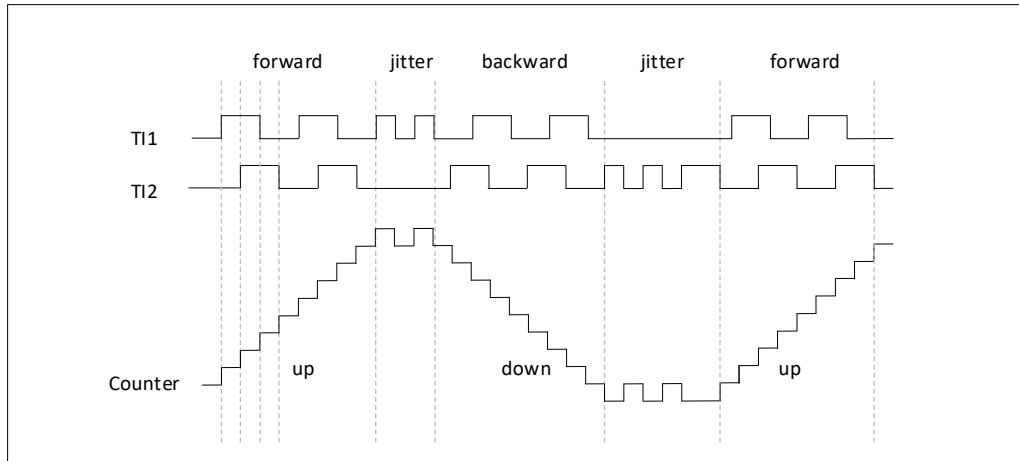
图 14-42 编码器模式下的计数器操作实例
