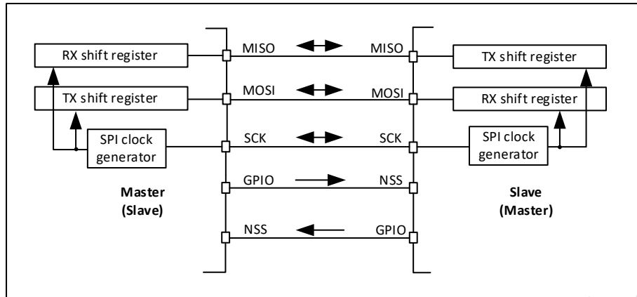
图 19-6 Multi-主机应用
