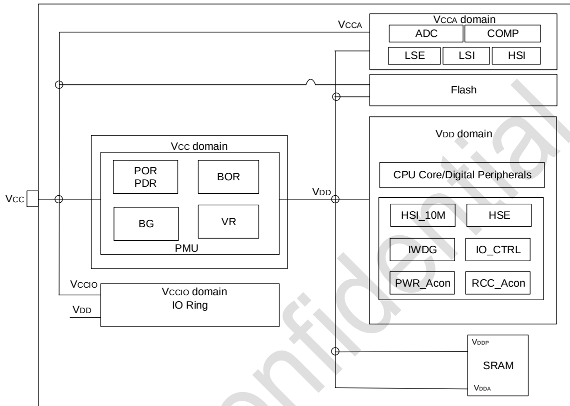
图 5-1 电源框图
