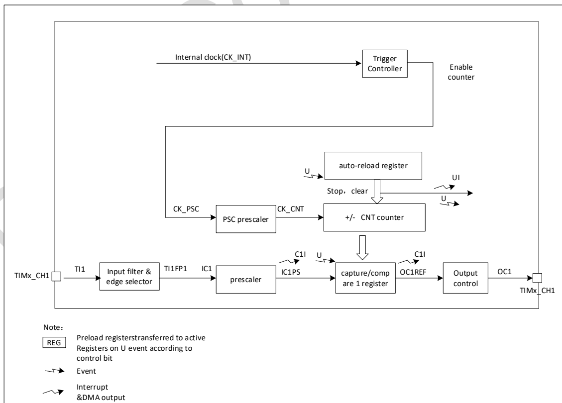
图 15-1 TIM14 架构框图
