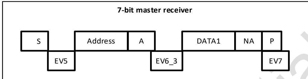
图 18-9 方法 2: N=1 时主模式发送时的时序
