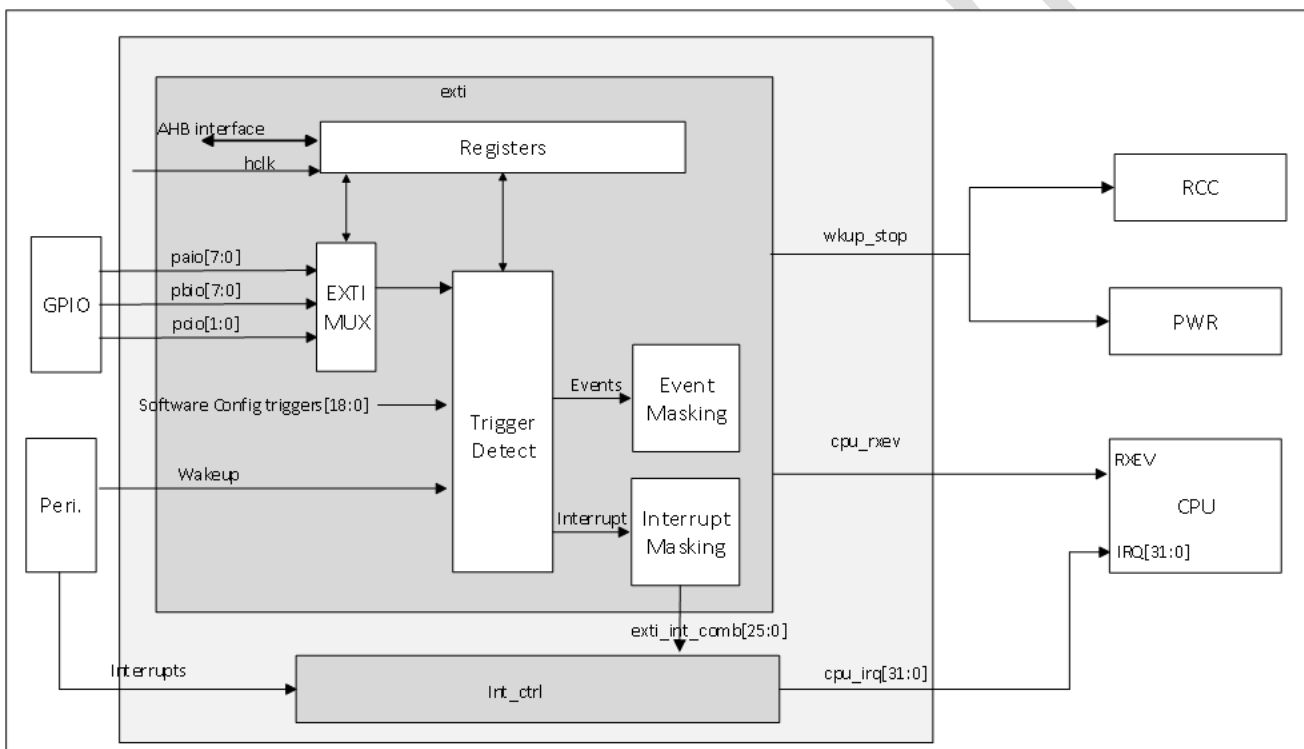
图 10-1 EXTI 框图
