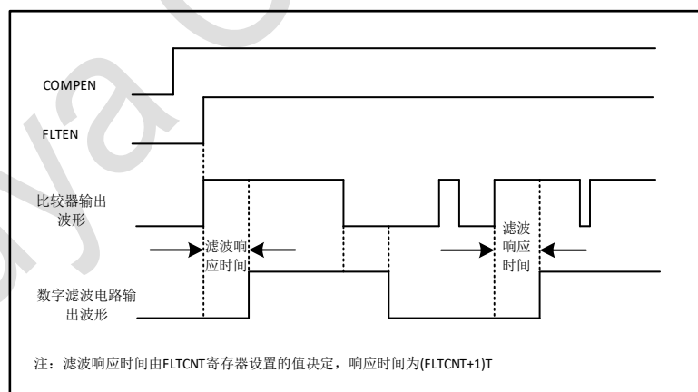
图 13-3 比较器滤波
