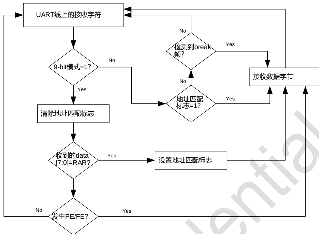
错误!链接无效。 图 20-6 硬件地址匹配接收模式
