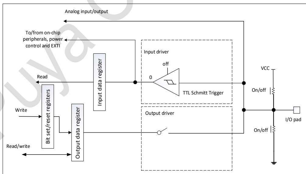
图 8-5 高阻抗模拟配置
