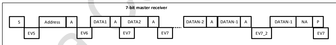
图 18-7 方法 2: N&gt;2 时主模式发送时的时序
