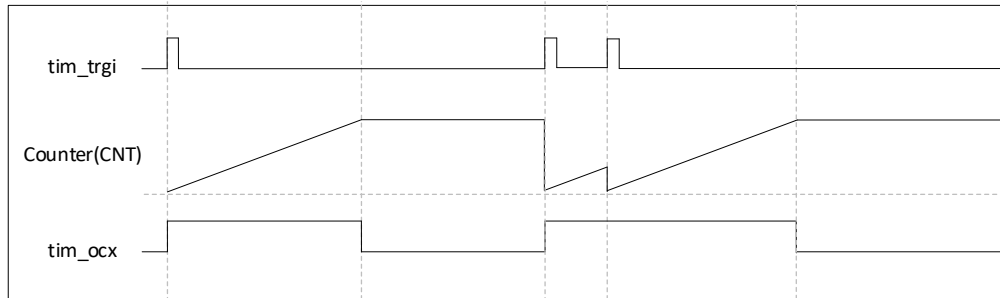
图 14-44 可重新触发单脉冲模式的示例
