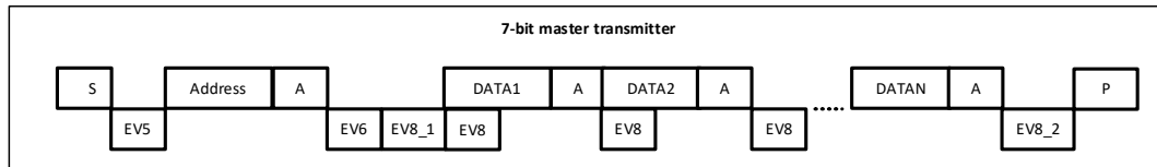
图 18-5 主发送器传送序列图
