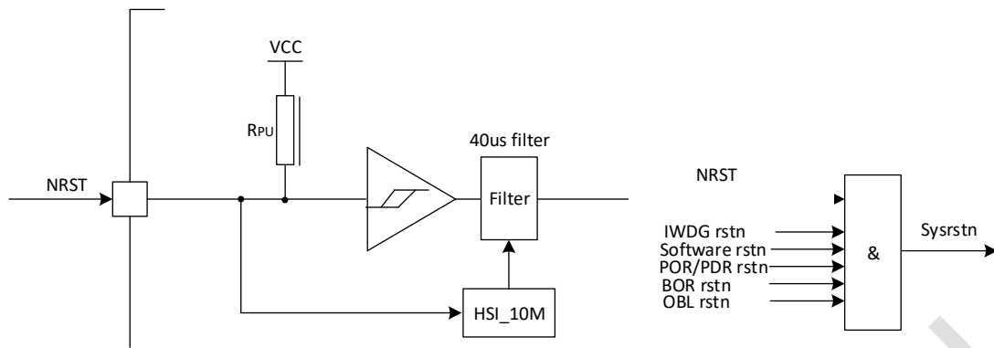
图 6-1 复位电路简化图
