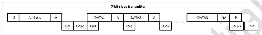
图 18-3 从发送器的传送序列图
