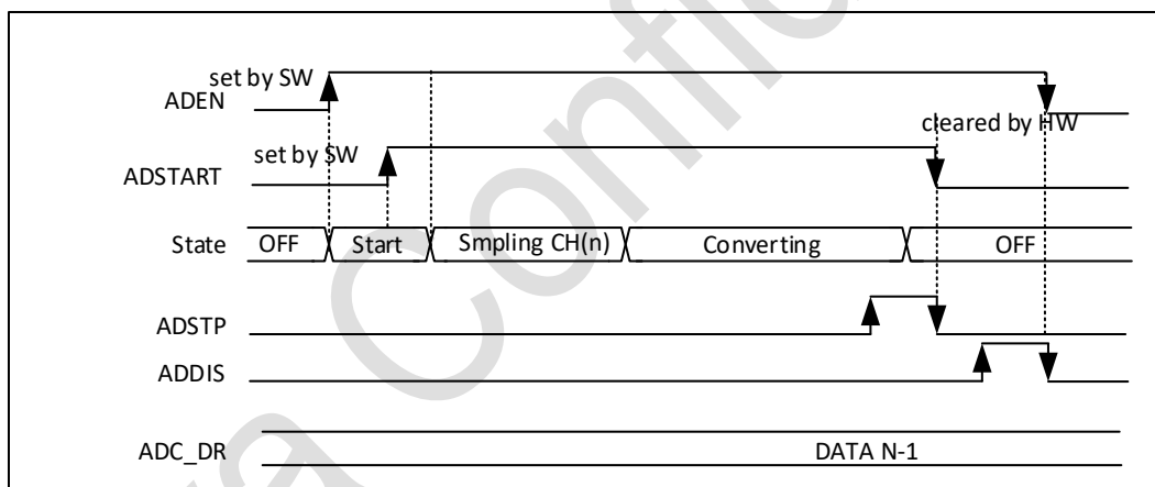
图 12-6 ADDSI 时序
