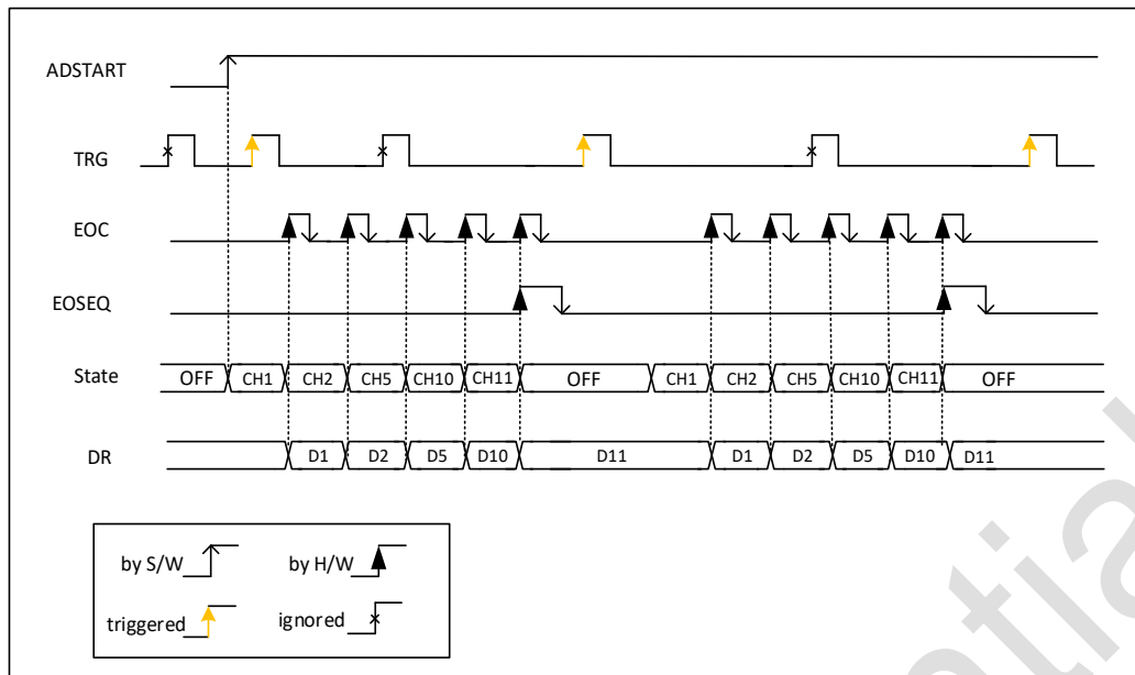
图 12-9 序列的单次转换, 硬件触发
