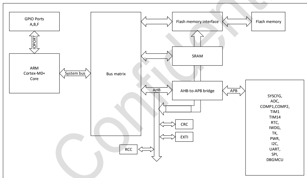
图 3-1 系统架构
