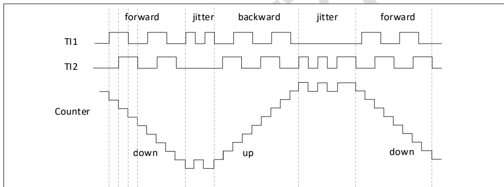
图 14-43 TI1P1 极性反转的编码器接口模式示例
