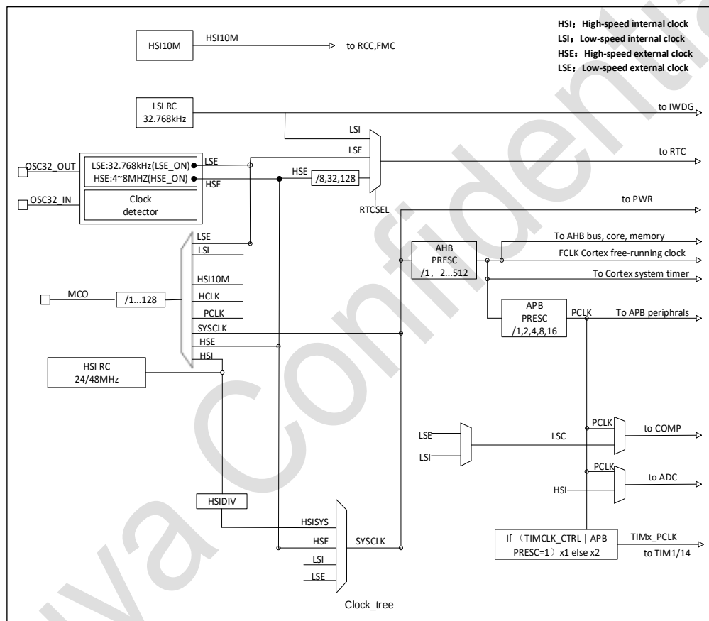
图 7-1 系统时钟结构图
