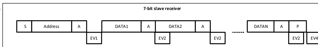
图 18-4 从接收器的传送序列图
