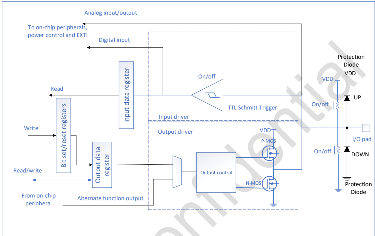
图 8-1 IO 端口位的基本结构
