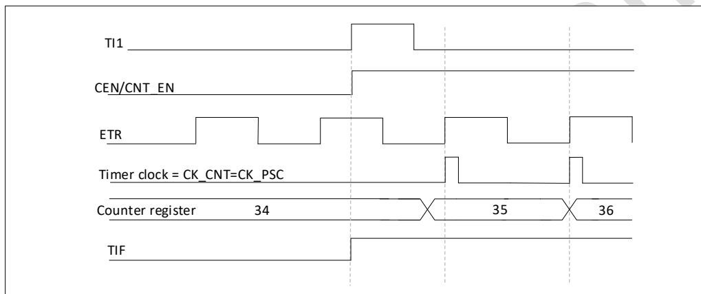
图 14-49 外部时钟模式 2 + 触发模式下的控制电路
