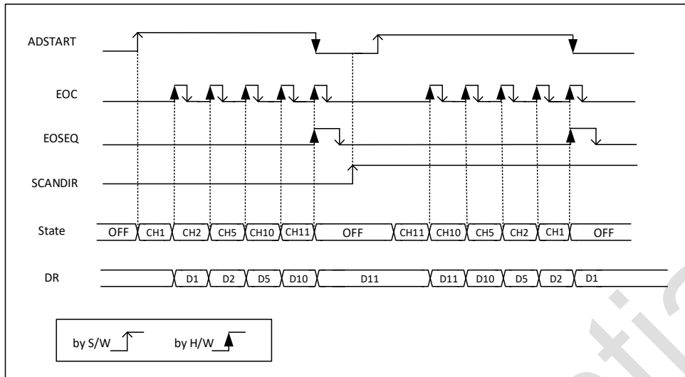
图 12-7 序列的单次转换, 软件触发
